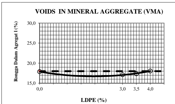
Gambar 7. Grafik Hubungan LDPE dan Voids In Mineral Agregate VMA
