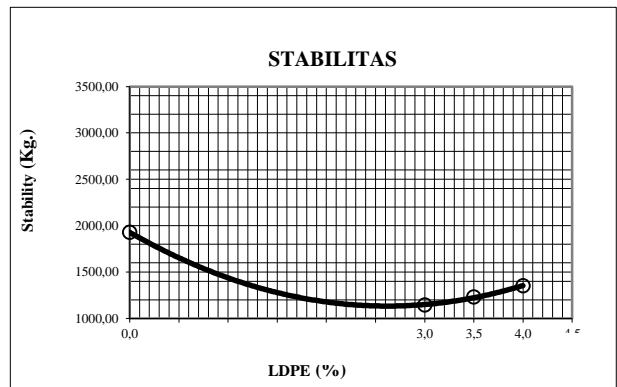
Gambar 2. Grafik Hubungan LDPE dan Stabilitas
