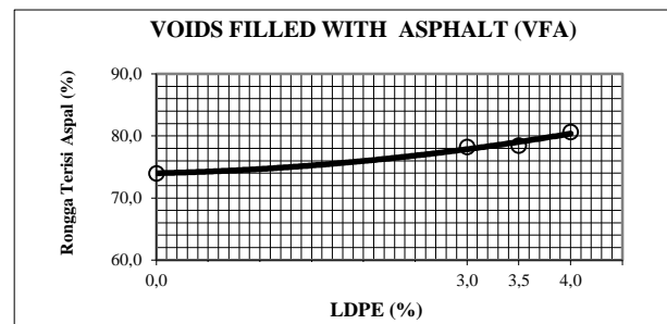
Gambar 8. Grafik Hubungan LDPE dan VFB
