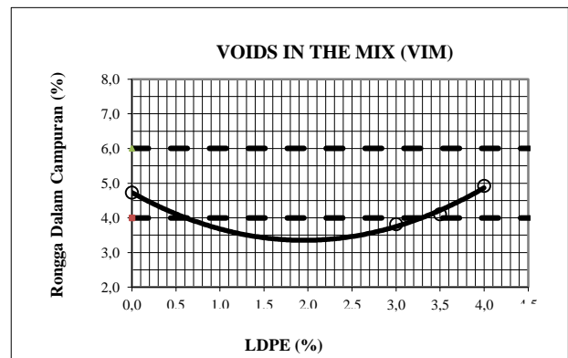
Gambar 6. Grafik Hubungan LDPE dan Voids In The Mix (VIM)
