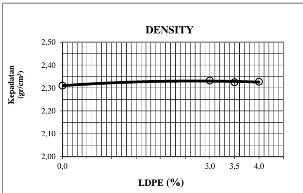
Gambar 5. Grafik Hubungan LDPE dan Kepadatan ( Density )
