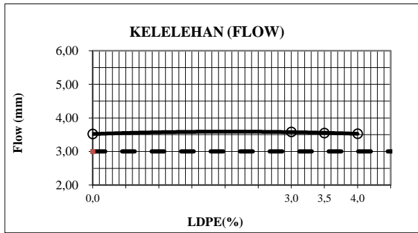
Gambar 3. Grafik Hubungan LDPE dan Kelelehan (Flow)
