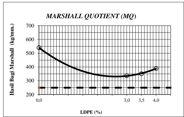
Gambar 4. Grafik Hubungan LDPE dan Marshall Quotient (MQ)
